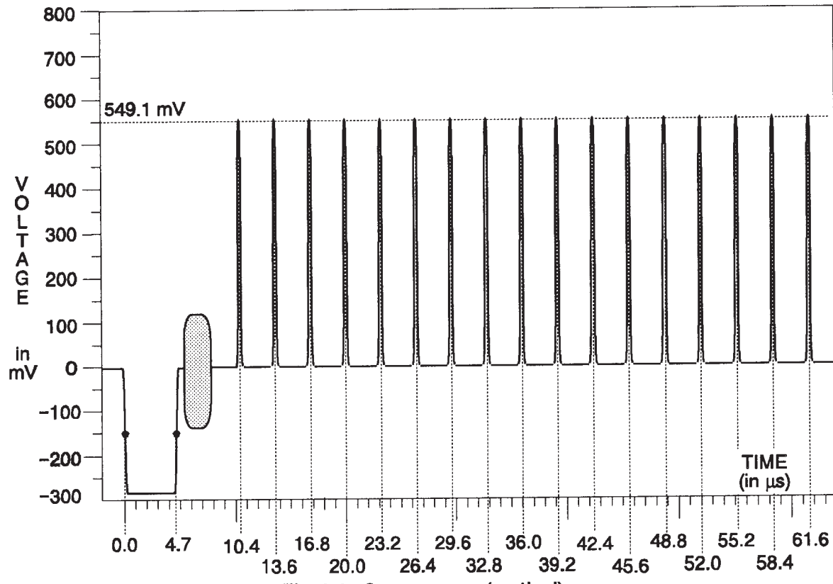
Fig. 3-6. Convergence (vertical).
