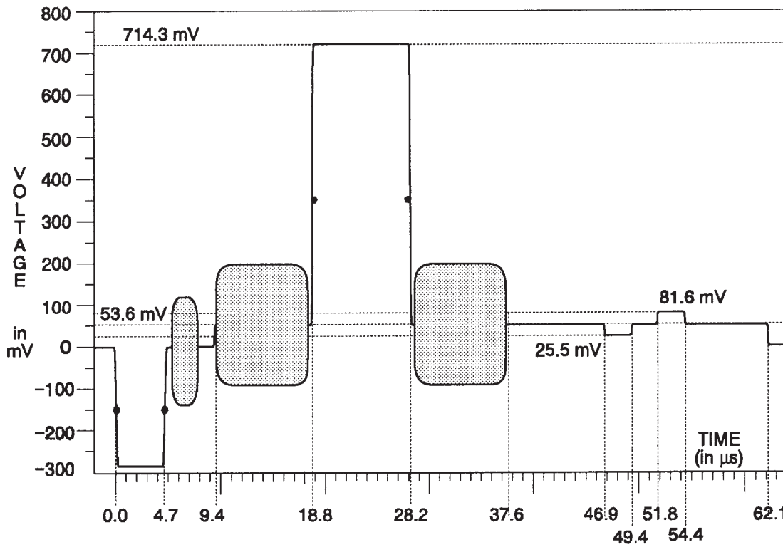
Fig. 3-4. SMPTE IYQB.
