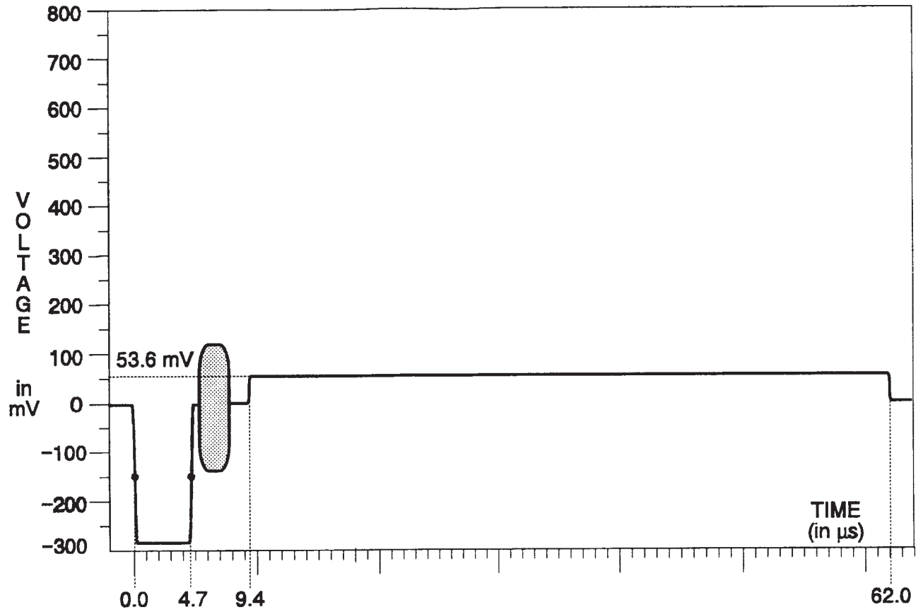
Fig. 3-16. Black Burst.
