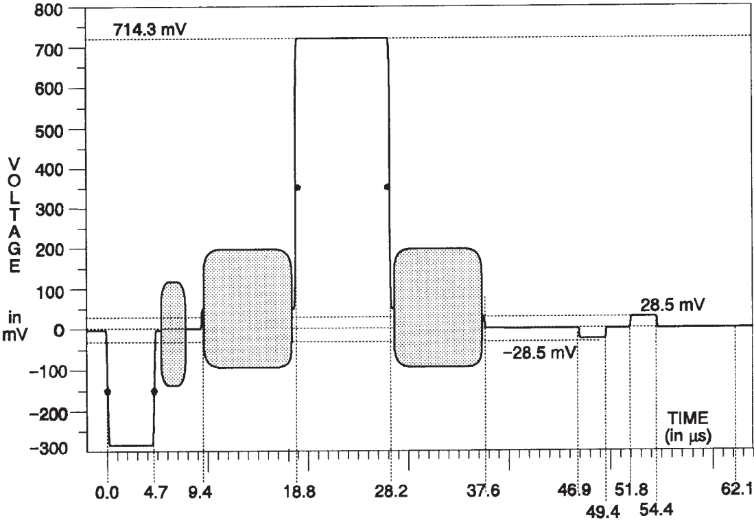
Fig. 6-3. SMPTE IYQB.
