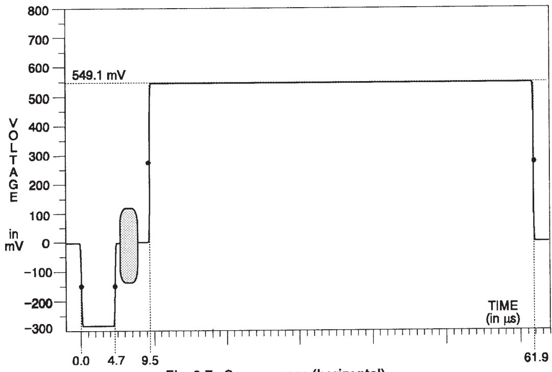
Fig. 3-7. Convergence (horizontal).
