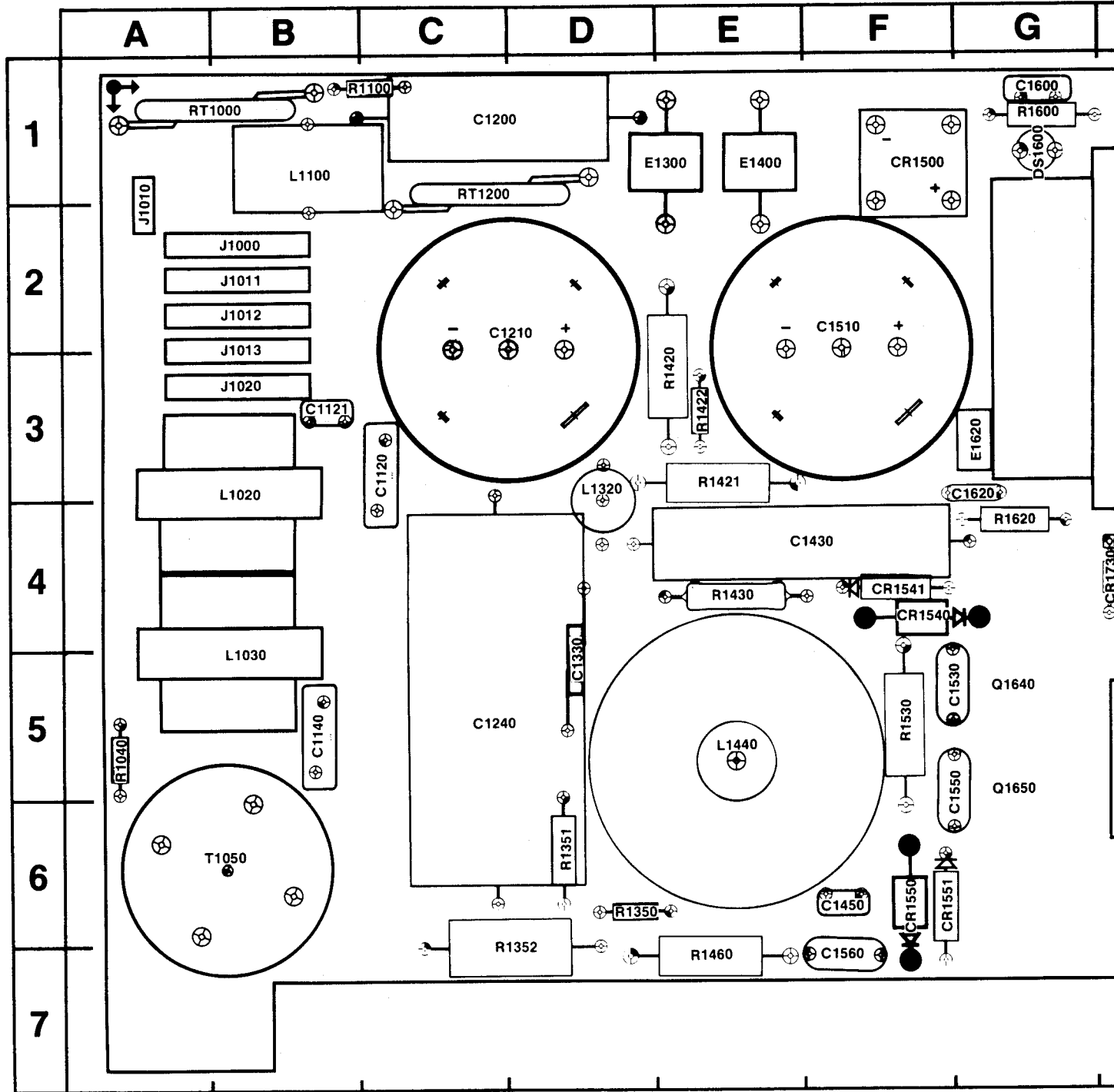
Fig. 8-1. Dc Power Suppl
