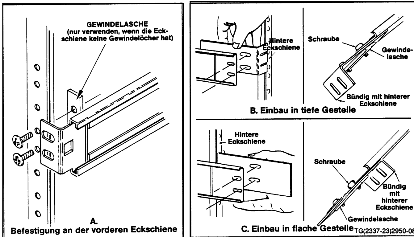
Bild 2-8. Gestelleinbau-Details.
