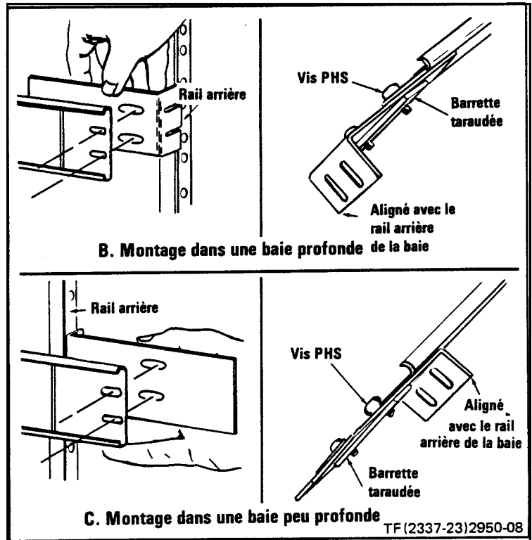
Fig. 2-8. Montage des rails à glissières sur la baie
