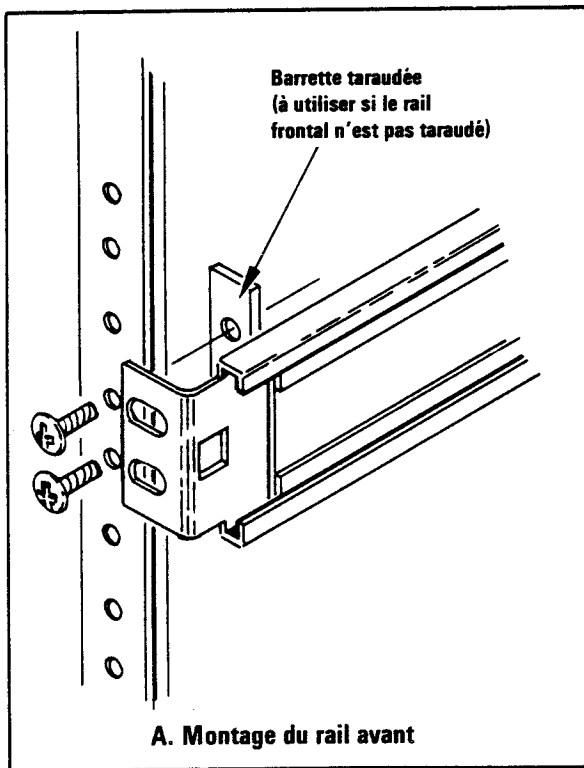
Fig. 2-8. Montage des rails à glissières sur la baie
