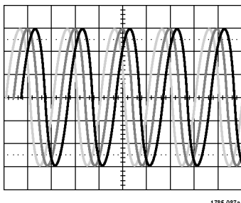
Untriggered display
