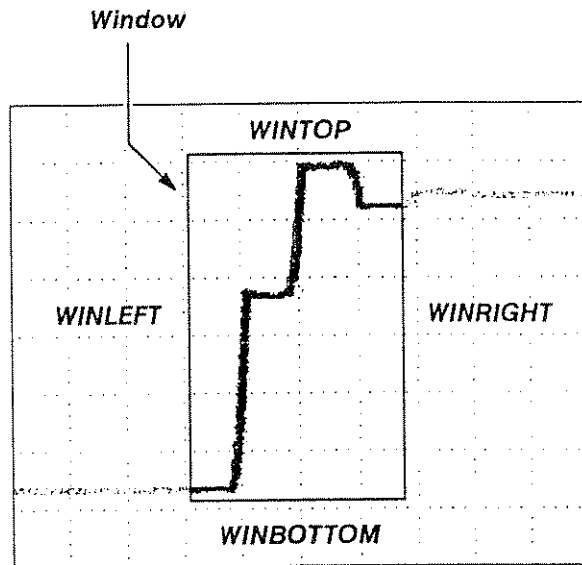
Histogram Window Parameters
