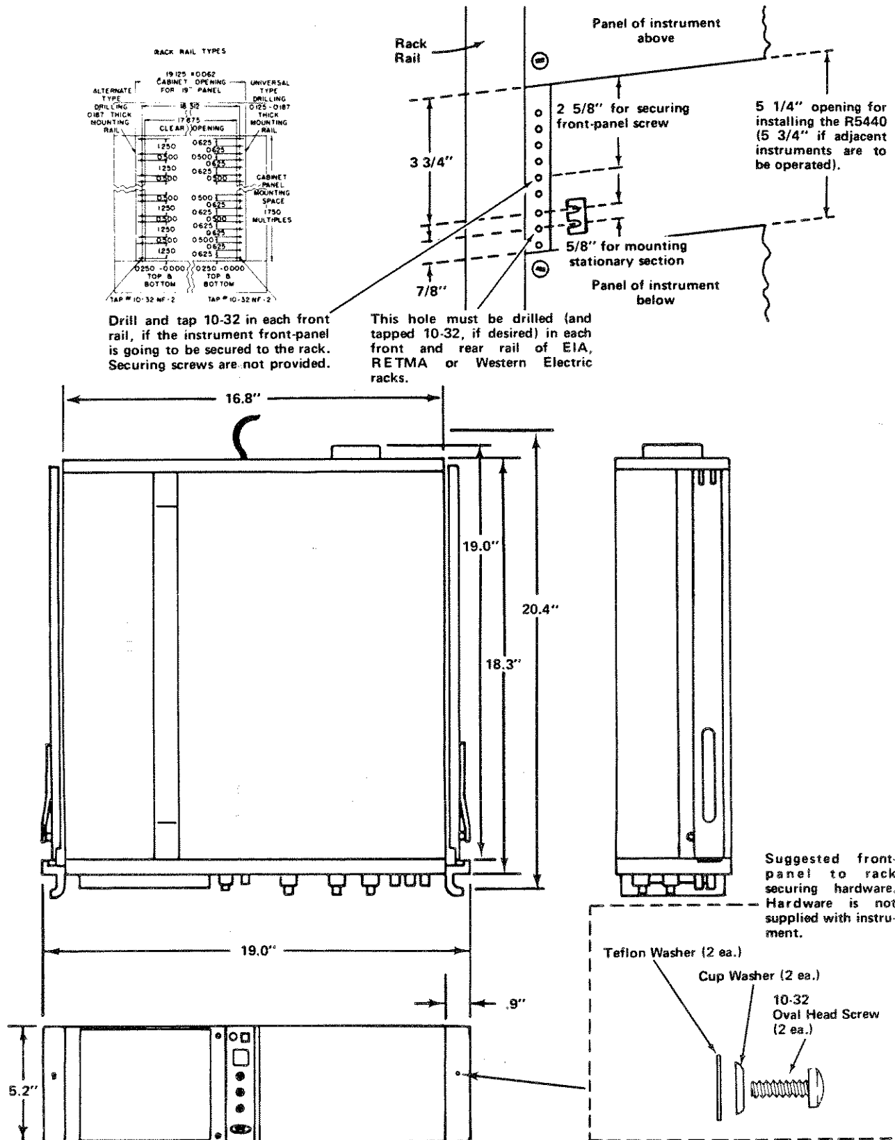
Fig. 1-5. Dimensional diagram.
