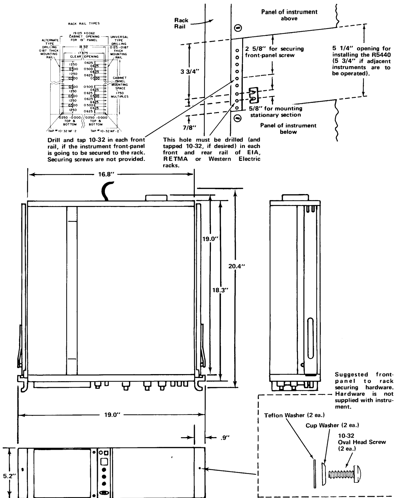
Fig. 1-5. Dimensional diagram.
