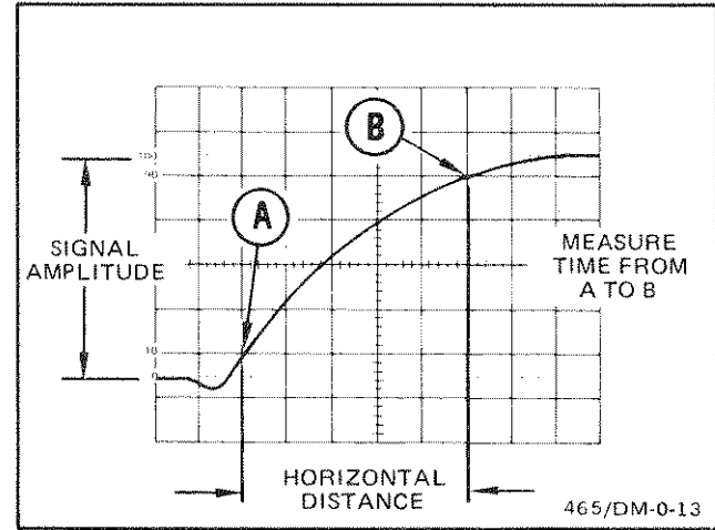
Fig. 19. Risetime.
