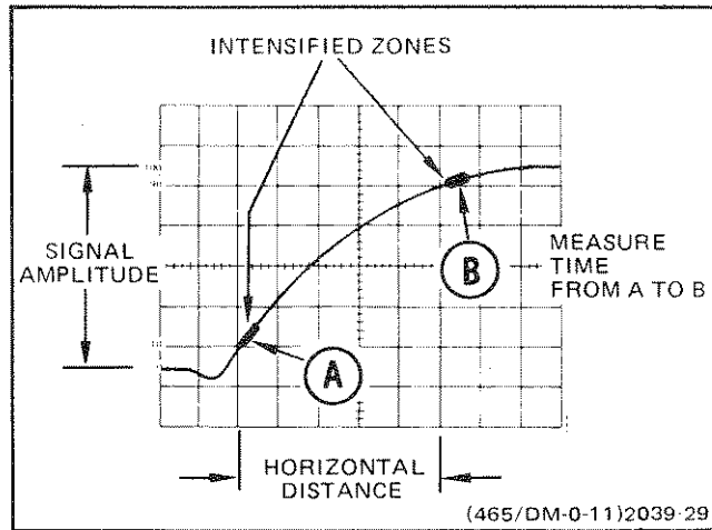
Fig. 28. Risetime.
