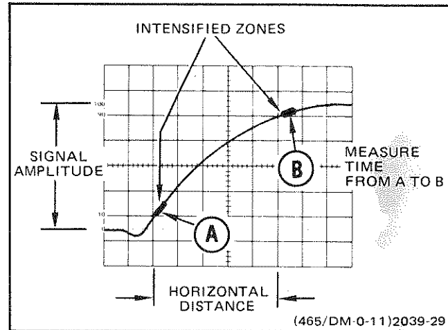
Fig. 32. Risetime.
