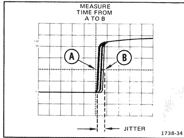
Fig. 23. Pulse jitter.
