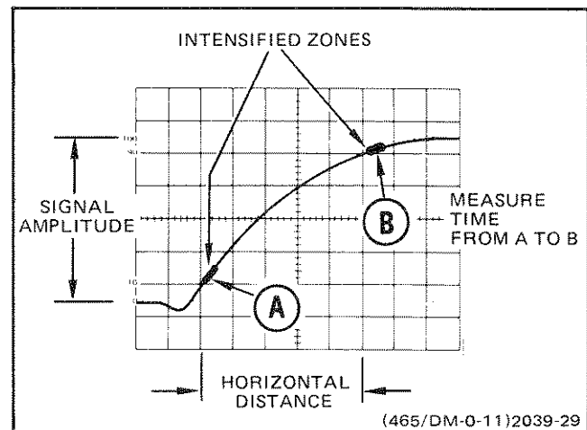
Fig. 32. Risetime.
