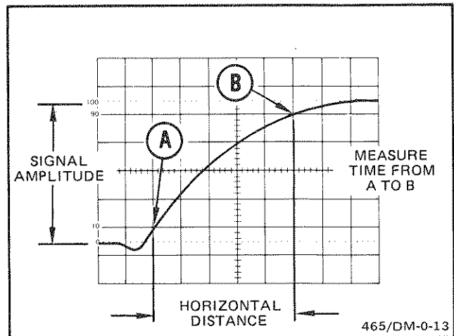
Fig. 19. Risetime.
