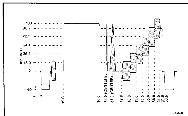
Fig. 6-23. NTC 7 Composite.
