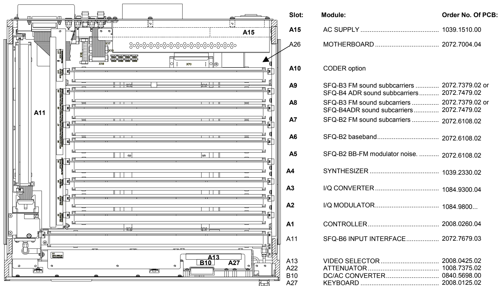
Fig. 1.5-2 Layout of modules
