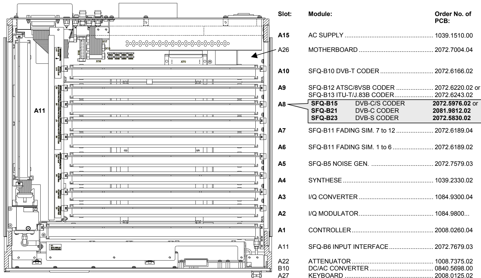
Fig. 1.5-4 Layout of modules
