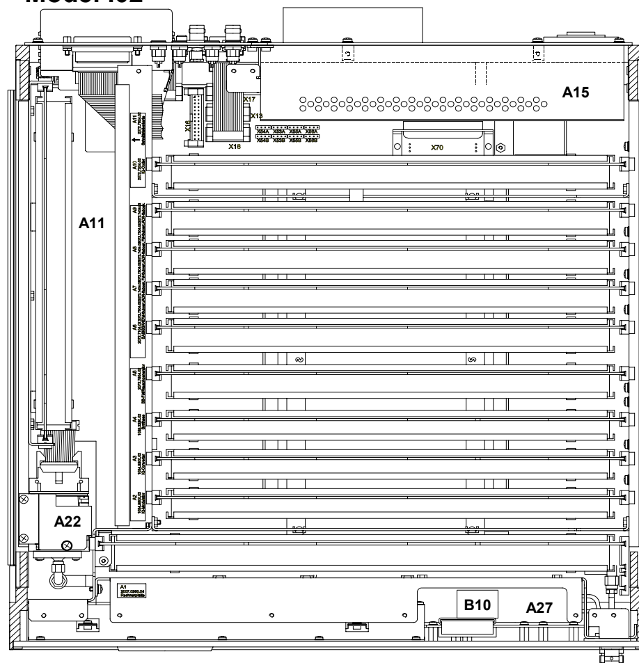
Fig. 1.5-1 Layout of modules
