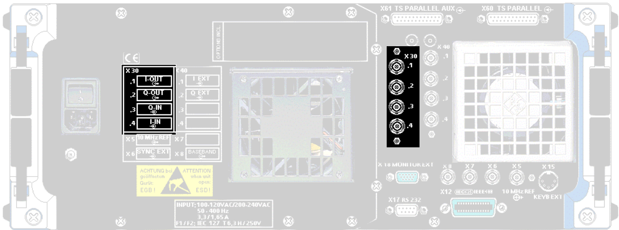
Fig. 1-9 SFQ-B14
