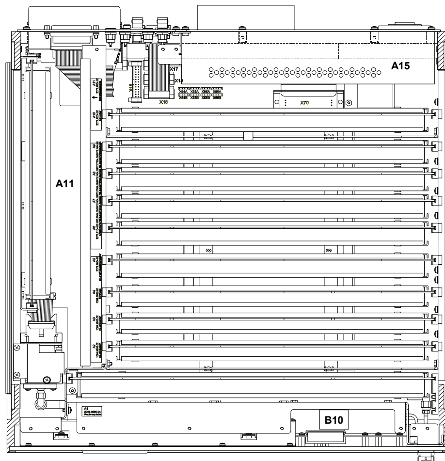
Fig. 1.5-3 Layout of modules
