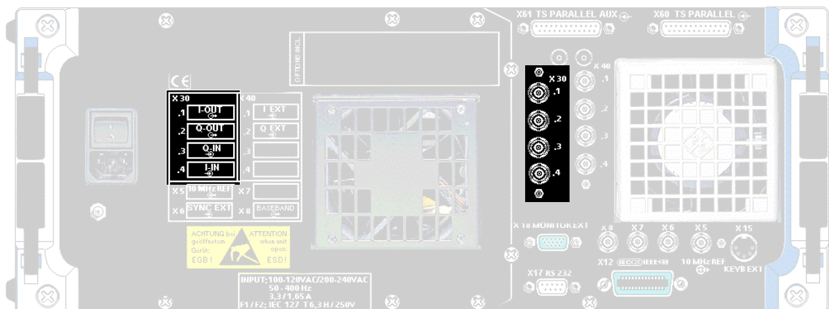
Fig. 1-10 SFQ-B27
