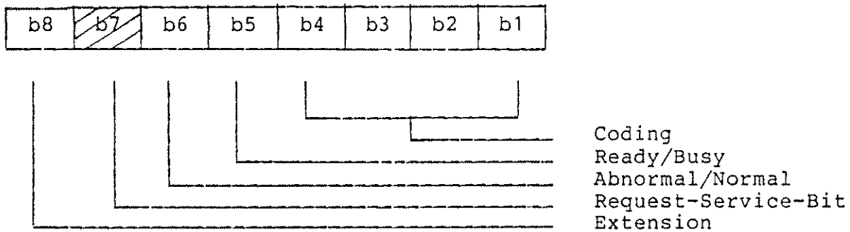
Fig. 2-14 Status byte
