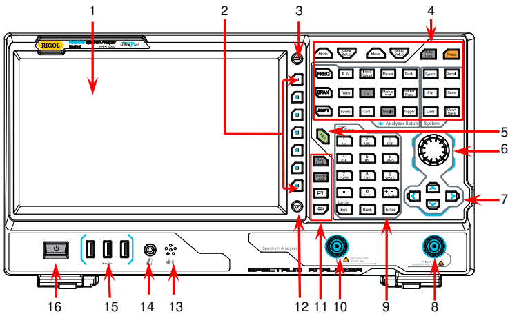
图 1 前面板
