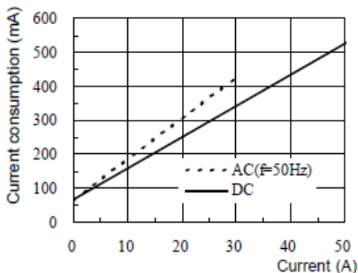
RP1004C
