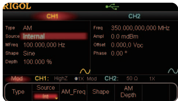
AM
