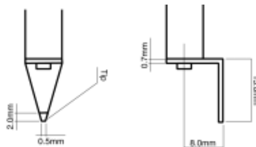
888-080 Dimensions
