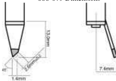
888-079 Dimensions
