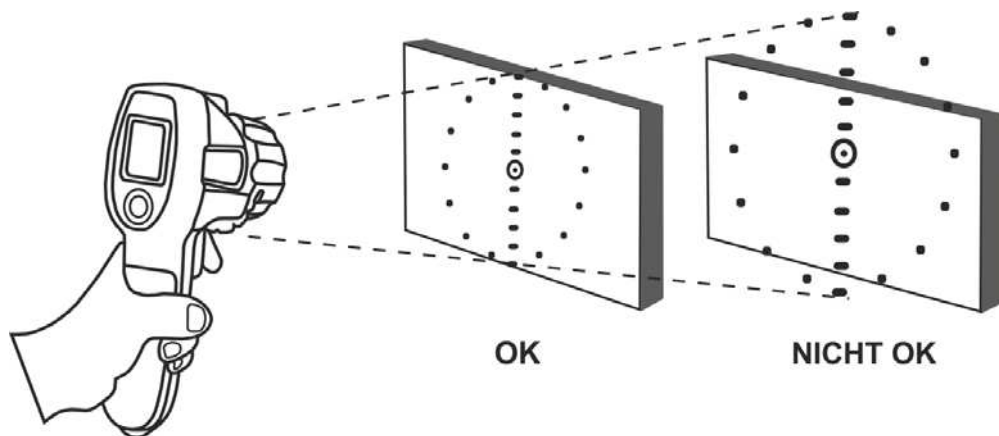
Abb. 17: Korrekte Messbedingungen
