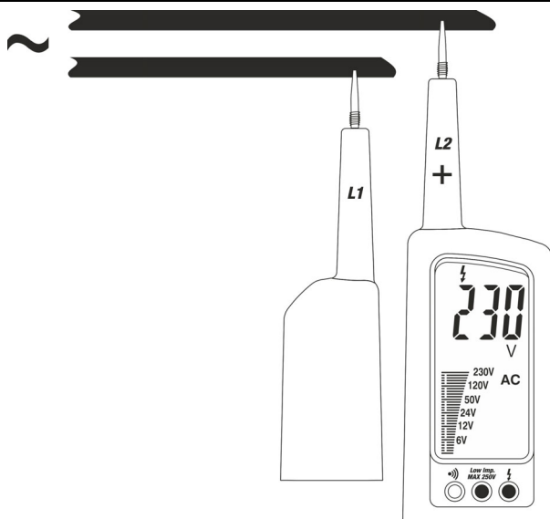
Fig. 4: Misura di Tensione AC con bassa impedenza
