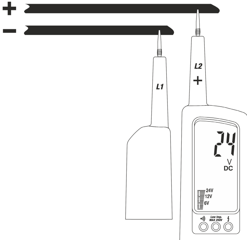
Abb. 2 DC Spannungsmessung
