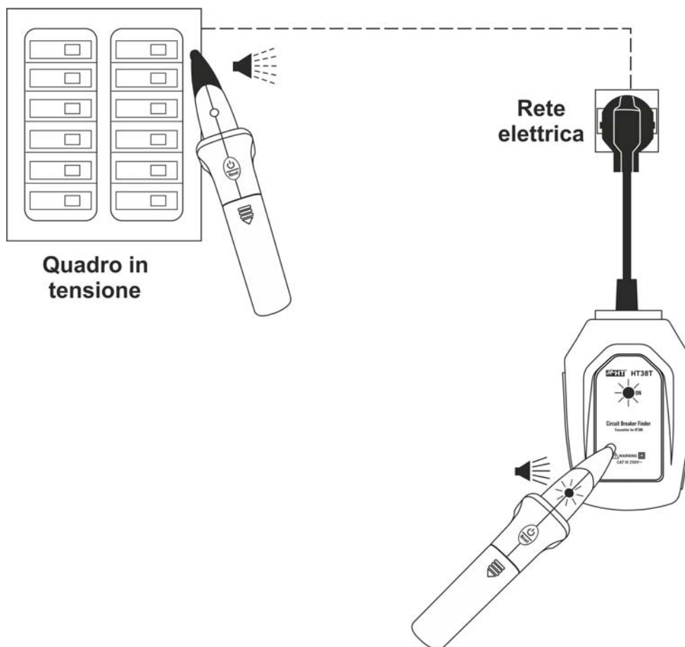
Fig. 3: Collegamento unità trasmettitore al circuito in prova
