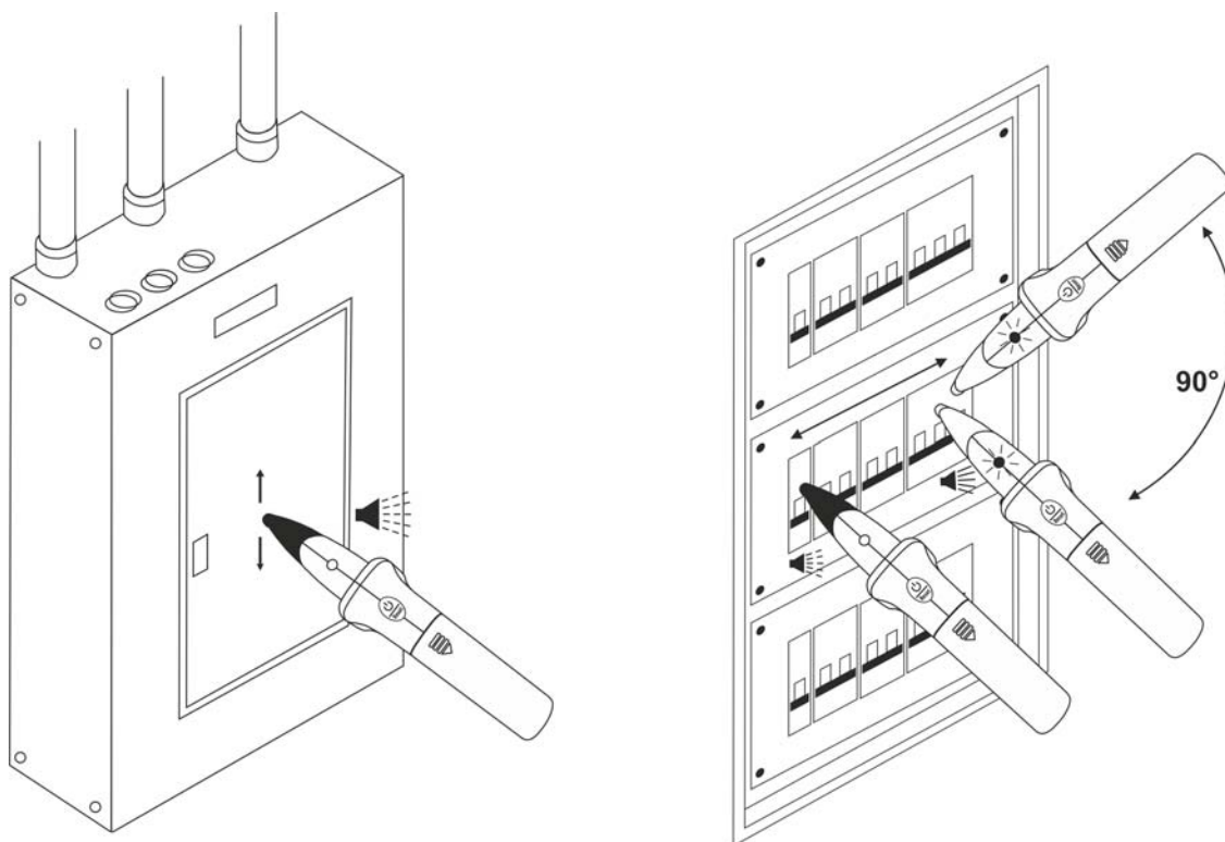
Fig. 4: Localizzazione del dispositivo di protezione
