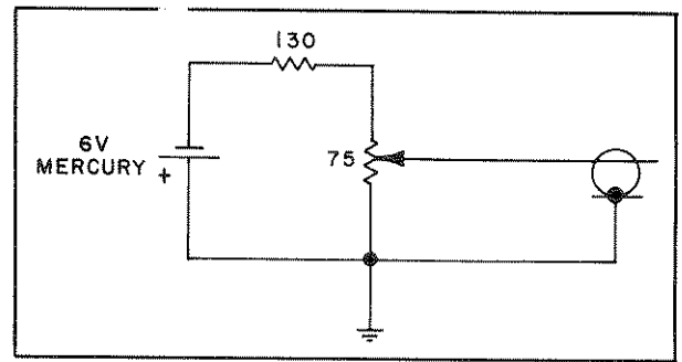
Figure 3-7. External VCO.
