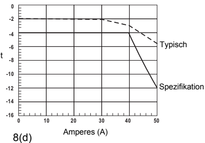
Abbildung 8(a – d): DC Signallinearität im Bereich von 0.1 V/A, typisch
