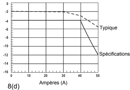
Figure 8(a – d): Linéarité pour Signal DC, gamme 0.1 V/A, typique
