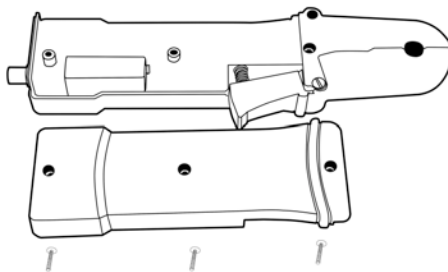
Abbildung 5: Einsetzen der Batterie
