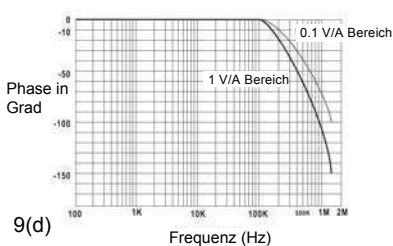
Abbildung 9(a - d): Phase gegen Frequenz bei Spitzenwert 1 A, typisch
