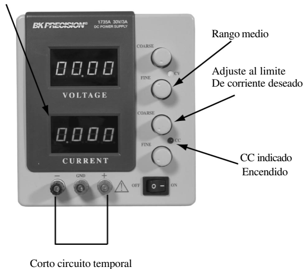
Figura 5. Estableciendo el limite de correinte
