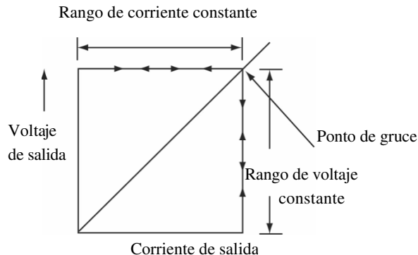
Figura 7. Voltaie constante/Corriente constante características
