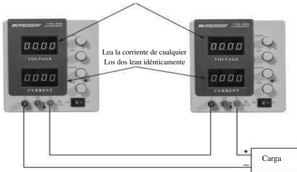
Figura 8 .Conectando dos fuentes de poder en serie
