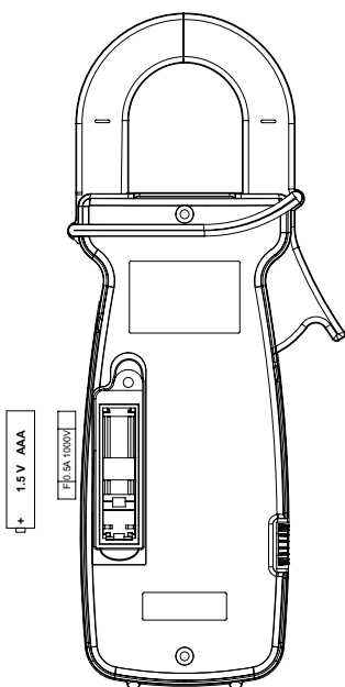
Fig 4. Batterisäkring
