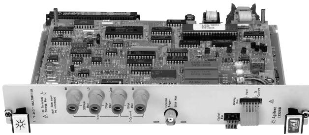
Agilent E1326B
