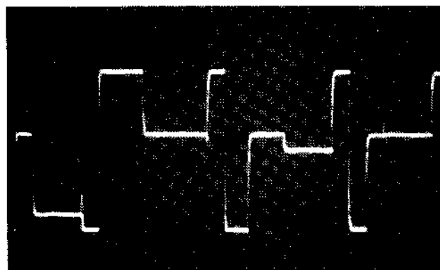
20ms/div. 0.5V/div.
