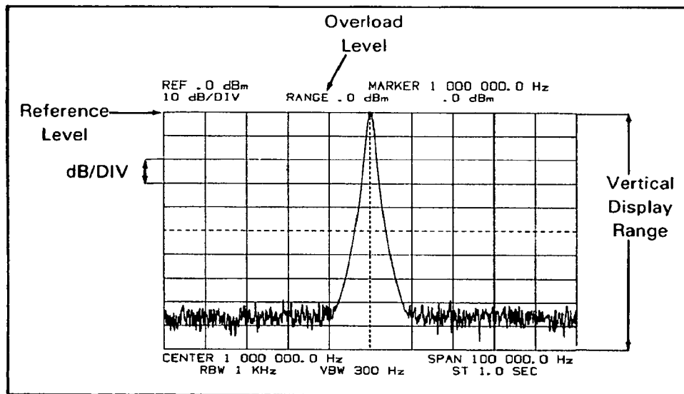
Amplitude Parameters
