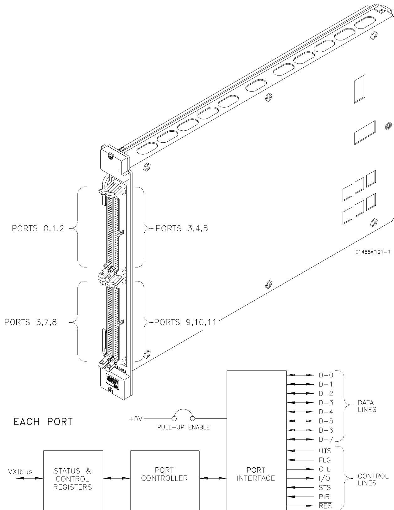
Figure 1-1. Agilent E1458A Digital I/O Module
